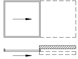
Schieber in Wandtasche oder Schieber vor Mauer
