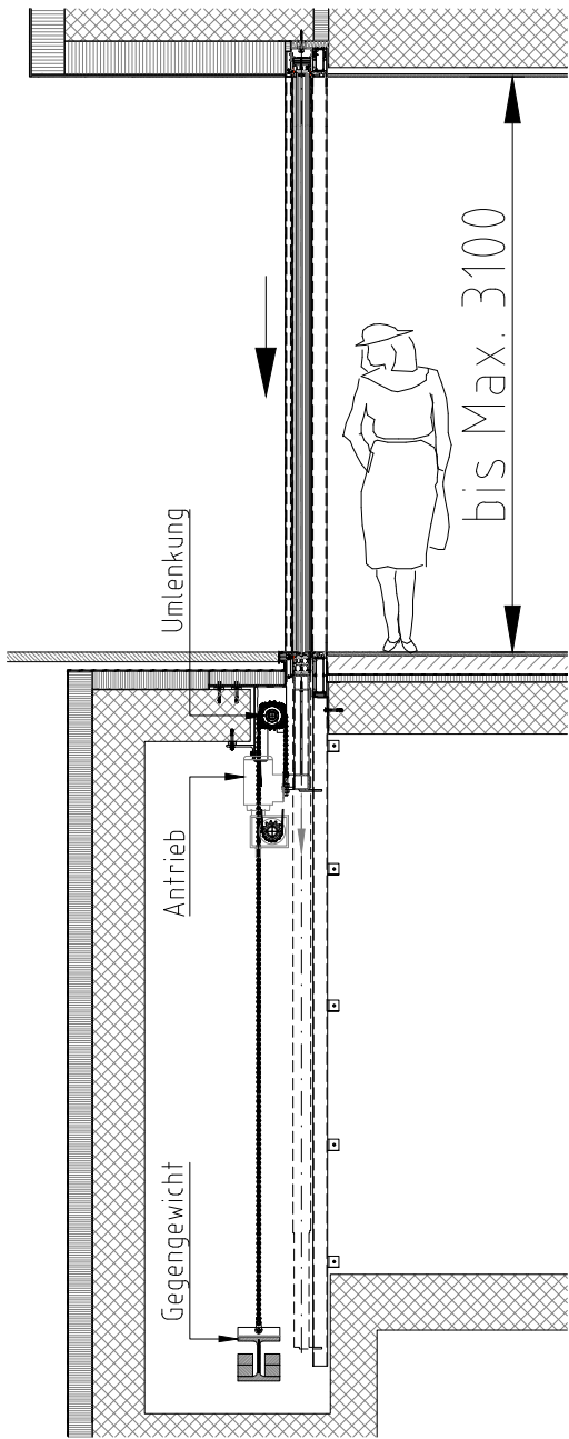
Vertikalschnitt
