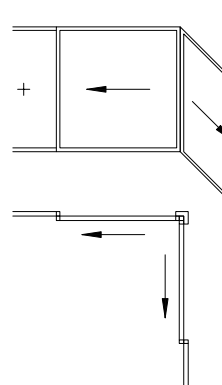
Angle interne avec montant
