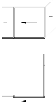
Angle externe avec montant
