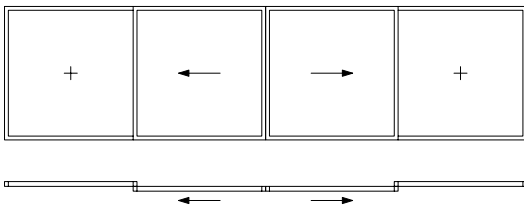
2 Flügel Mitte (Vertikalstoss mit Profilen)
