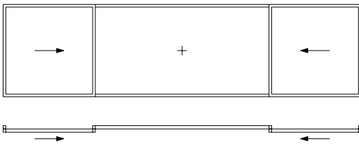
2 Flügel Aussen mit Festverglasung Mitte (Var.)
