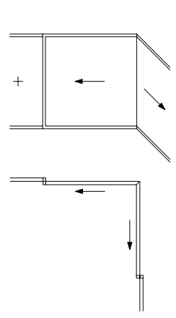
Innenecke Ganzglas
