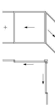
Innenecke mit Profil
